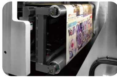
2 Web guide
